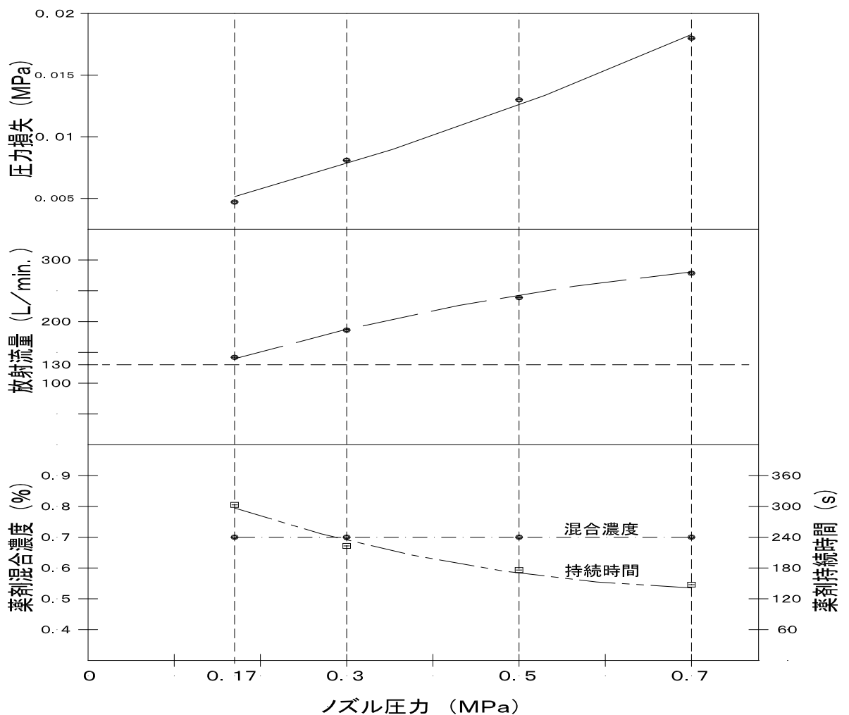
【圧力損失／放射流量／薬剤混合濃度・持続時間】グラフ
